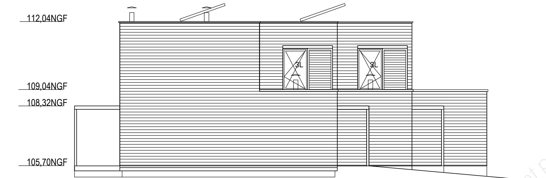
FACADE EST
